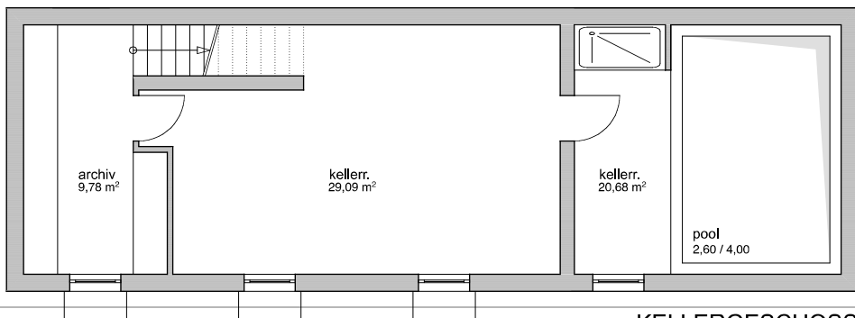
KELLERGESCHOSS
