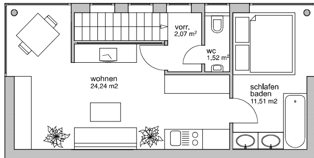
OBERGESCHOSS
