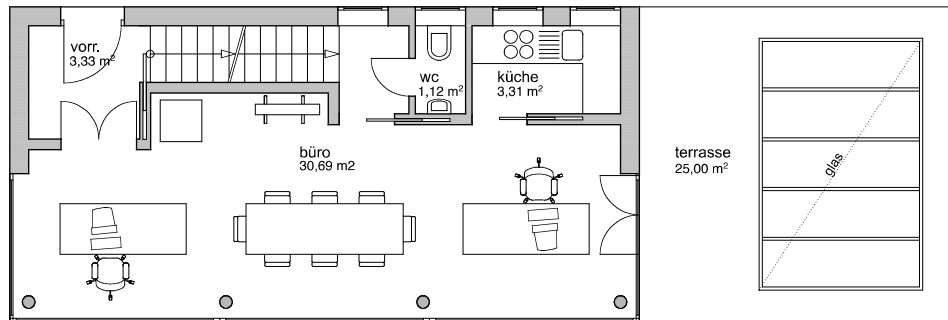
ERDGESCHOSS
