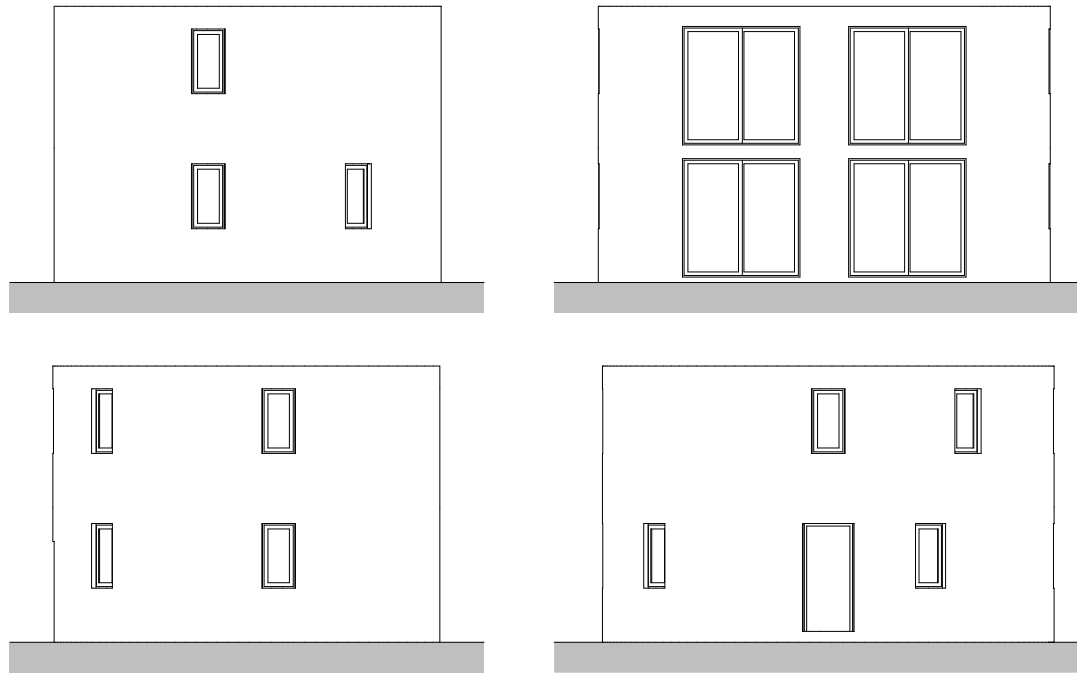
ANSICHTEN
