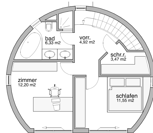
OBERGESCHOSS
