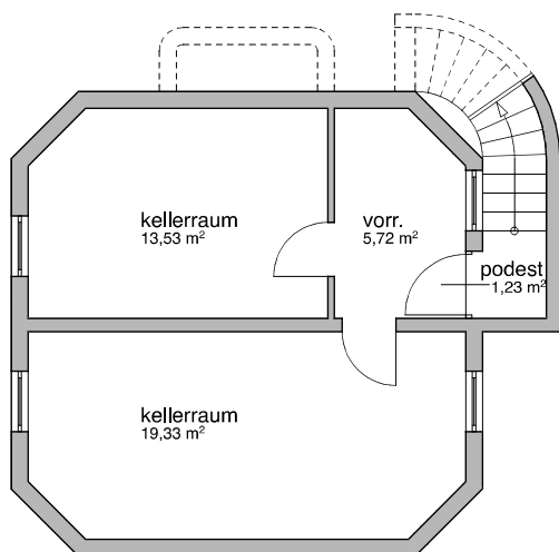
KELLERGECHOSS
