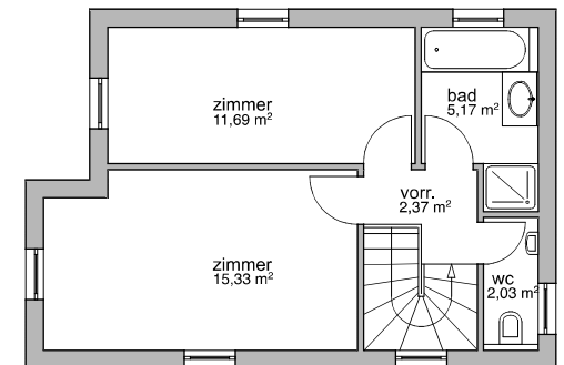
OBERGECHOSS
