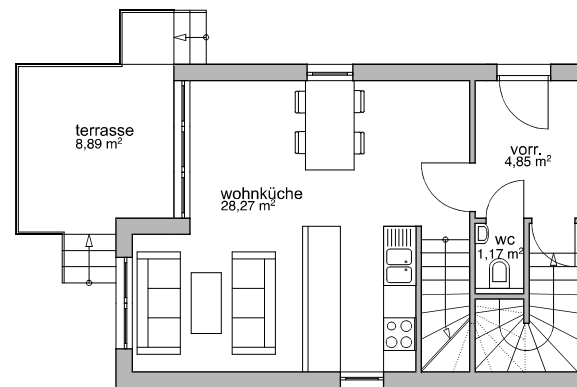
ERDGECHOSS
