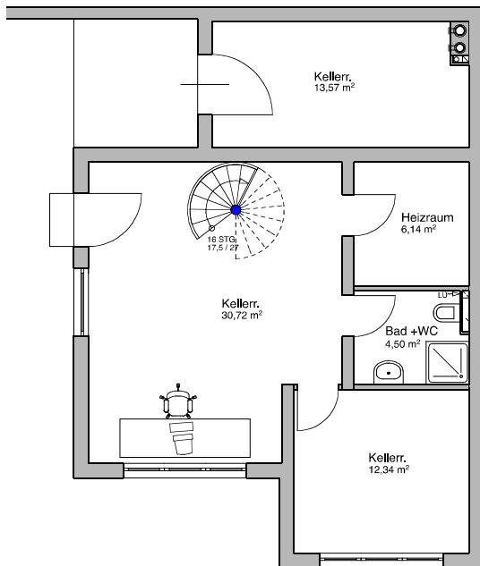
KELLERGESCHOSS
