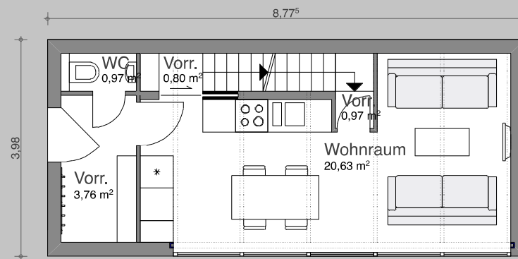
erdgeschoss
