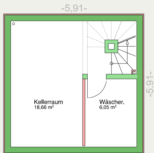
KELLERGECHOSS
