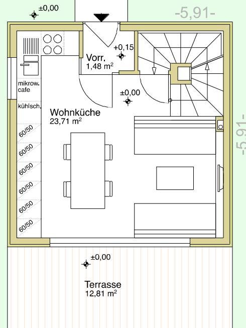
ERDGESCHOSS
