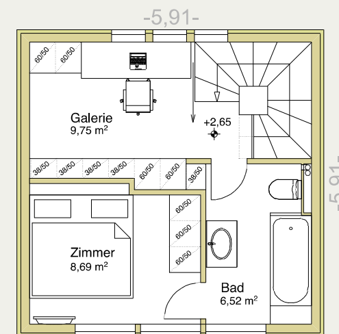
OBERGESCHOSS
