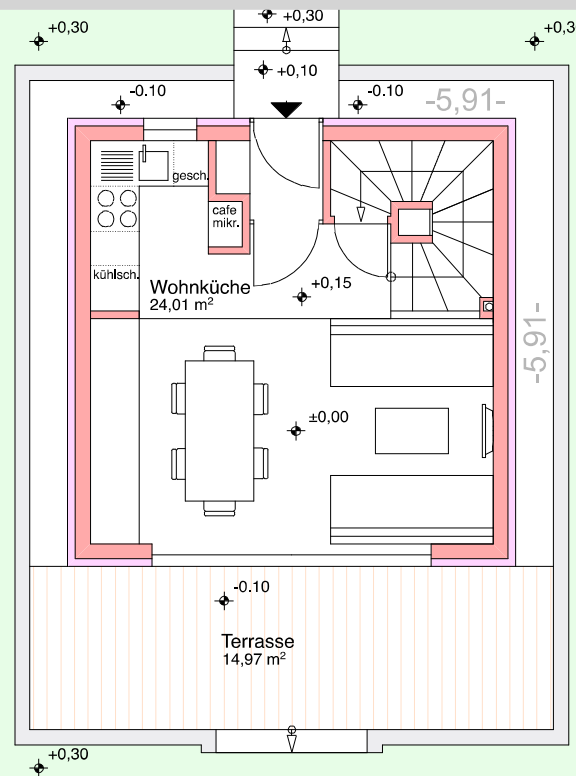
ERDGESCHOSS
