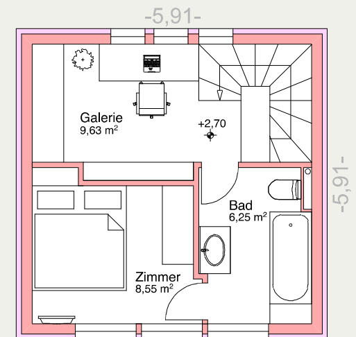
OBERGESCHOSS
